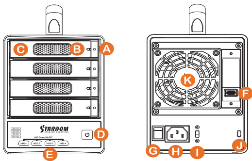
前視圖
